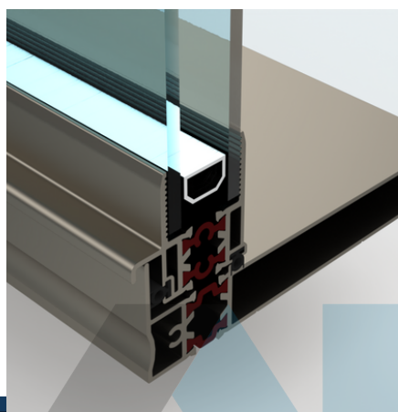
Detalj donjeg dela sa izolacijom Bottom case detail with barrier
