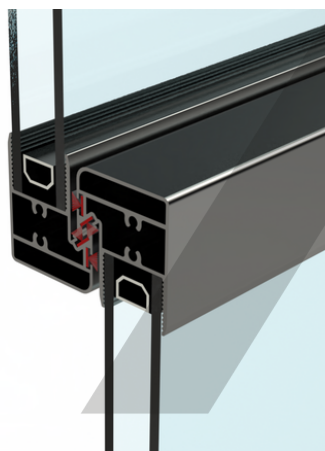
Izolovani spoj sa stegom Clamp joint
