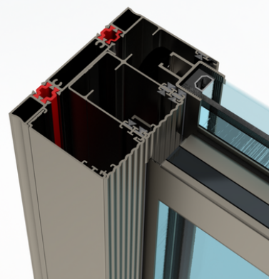
Detalj izolovanog bočnog okvira Side frame detail with barrier
