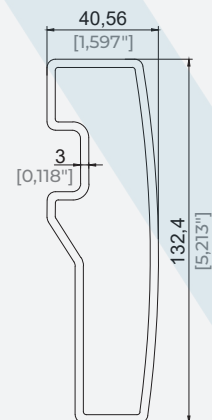
40,6x132,4 Veza profila oluka 40,6x132,4 Gutter Profile Connection
