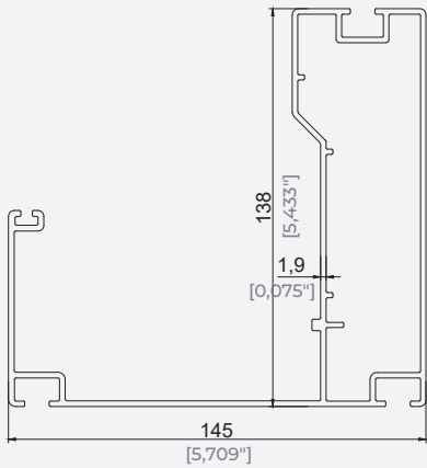
145x138 Oluk Profil 145x138 Eco Gutter Profile
