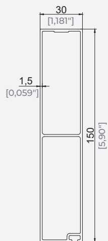
30x150 Kutni Profil 30x150 Box Profile
