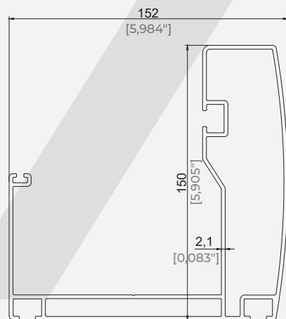
152x150 Oluk Profil 152X150 Gutter Profili
