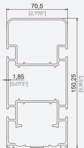
70,5 x 150,25 Šine Profil 70,5 x 150,25 Rail Profile
