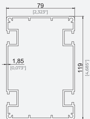
Horizontalni Profil Horizontal Profile
