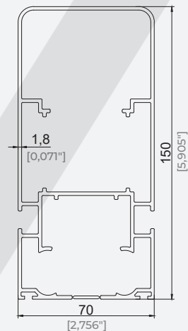
70x150 Šine Profil 70x150 Eco Rail Profile
